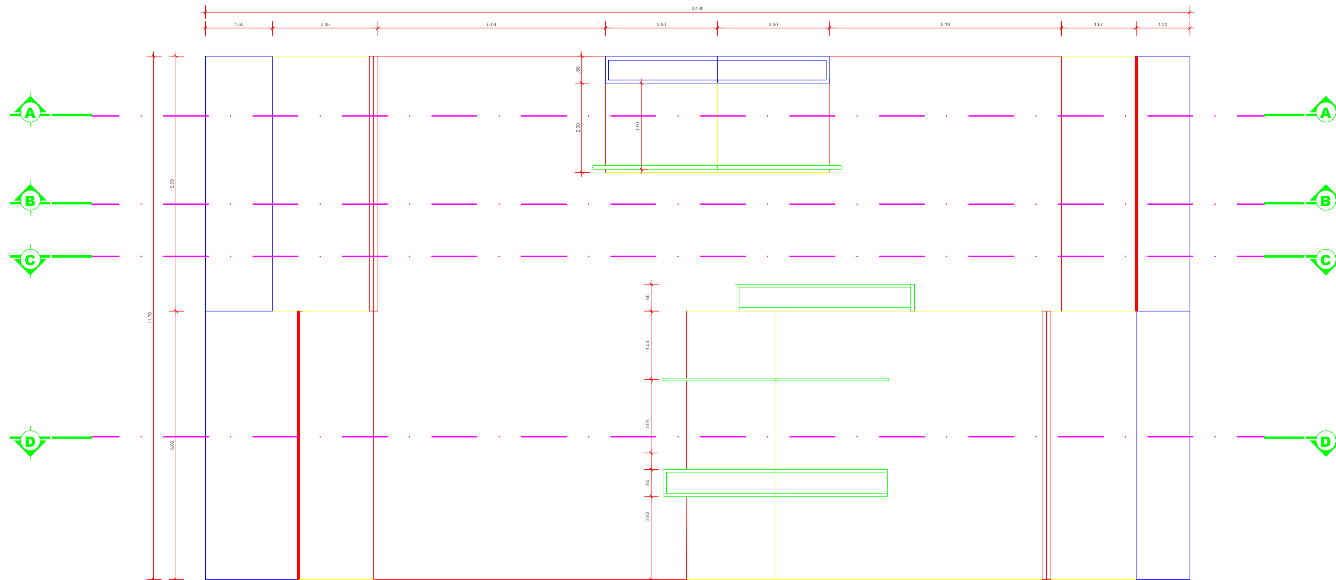
PLANTA BAIXA ESC. 1:50
